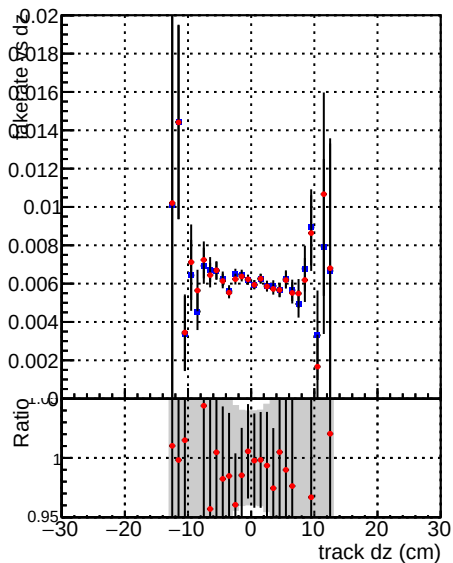
—●— DQM_mkFit_XiMinusNOPU_newDefault5 —●— DQM_mkFit_XiMinusNOPUold-lowlpt
