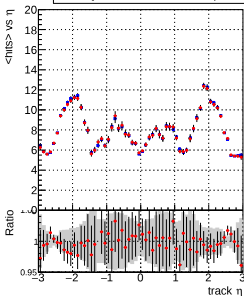
— DQM_mkFit_XiMinusNOPU_newDefault5 — DQM_mkFit_XiMinusNOPUold-lowpt
