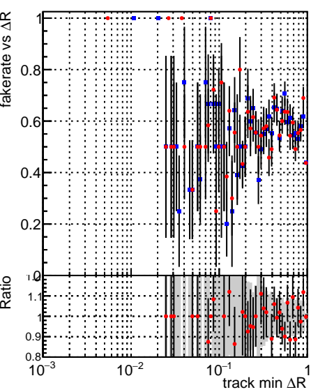
Fake rate vs \Delta R(\text{track, jet}) —■— DQM_mkFit_XiMinusNOPU_newDefault5 —●— DQM_mkFit_XiMinusNOPUold-lowpt
