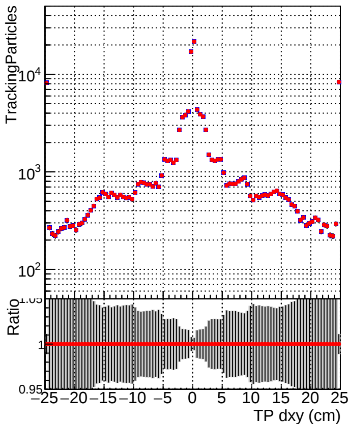
■ DQM_mkFit_XiMinusNOPU_newDefault5 ■ DQM_mkFit_XiMinusNOPUold-lowpt
