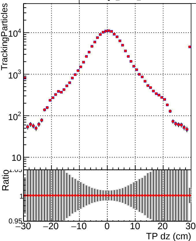
■ DQM_mkFit_XiMinusNOPU_newDefault5 ■ DQM_mkFit_XiMinusNOPUold-lowpt
