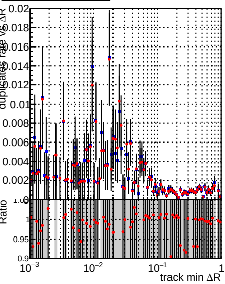
Legend: \blacksquare DQM_mkFit_XiMinusNOPU_newDefault5 \bullet DQM_mkFit_XiMinusNOPUold-lowpt
