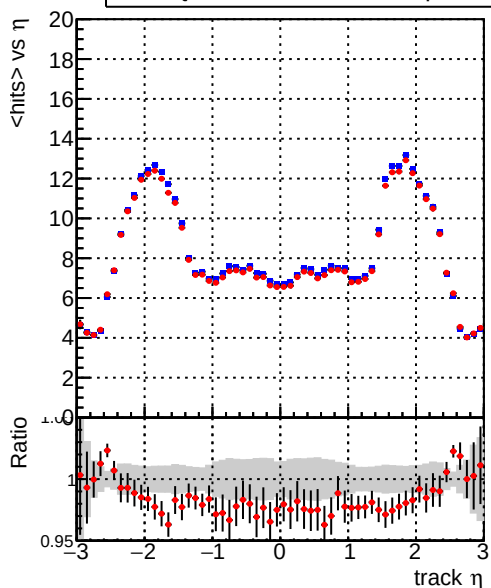
— DQM_mkFit_XiMinusNOPU_newDefault5 — DQM_mkFit_XiMinusNOPUold-lowpt mean hits vs \eta
