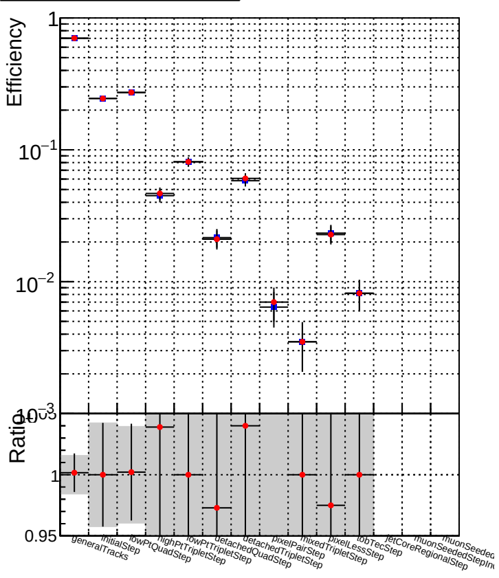
DQM_mkFit_XiMinusNOPU_newDefault5 DQM_mkFit_XiMinusNOPUold-lowpt
