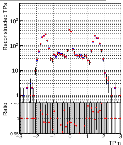
—•— DQM_mkFit_XiMinusNOPU_newDefault5 —•— DQM_mkFit_XiMinusNOPUold-lowpt
