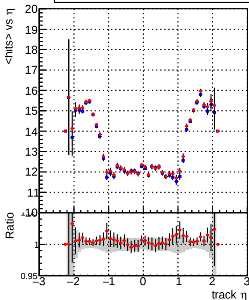
mean hits Legend: — DQM_mkFit_XiMinusNOPU_newDefault5, — DQM_mkFit_XiMinusNOPUold-lowpt
