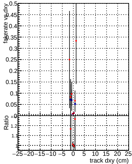
—●— DQM_mkFit_XiMinusNOPU_newDefault5 —●— DQM_mkFit_XiMinusNOPUold-lowpvt
