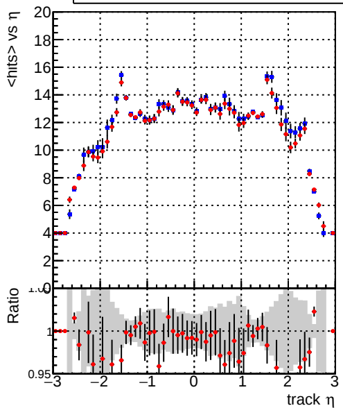
mean hits — DQM_mkFit_XiMinusNOPU_newDefault5 — DQM_mkFit_XiMinusNOPUold-lowpt
