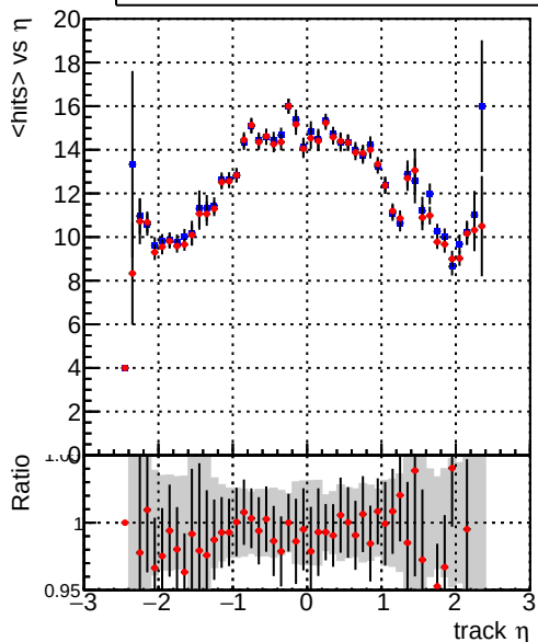
— DQM_mkFit_XiMinusNOPU_newDefault5 — DQM_mkFit_XiMinusNOPUold-lowpt mean hits
