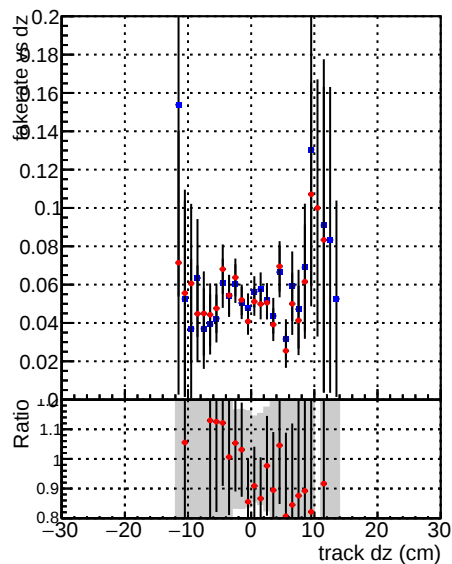
—●— DQM_mkFit_XiMinusNOPU_newDefault5 —●— DQM_mkFit_XiMinusNOPUold-lowpT
