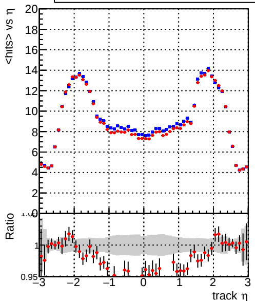
mean hits vs \eta — DQM_mkFit_XiMinusNOPU_newDefault5 — DQM_mkFit_XiMinusNOPUold-lowpt
