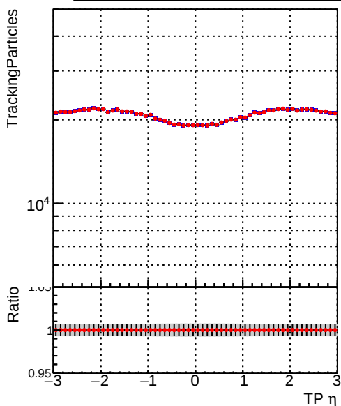
—•— DQM_mkFit_XiMinusNOPU_newDefault5 —•— DQM_mkFit_XiMinusNOPUold-lowpt
