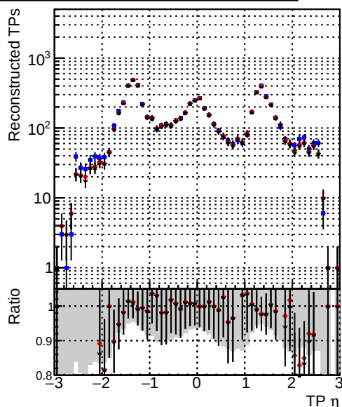
—•— DQM_mkFit5_XiMinusNOPUold-lowpt —•— DQM_mkFit5_XiMinusNOPU_newDefault5 —•— DQM_mkFit5_XiMinusNOPU_NEWdefault_specPLeSS3
