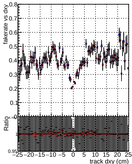
— DOM mkFit5 XiMinusNOPUold-lowpt — DOM mkFit XiMinusNOPU newDefault5 — DOM mkFit XiMinusNOPU Newdefault specPless3
