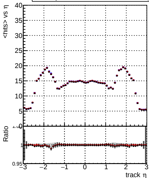
mean hit — DQM_mkFit5_XiMinusNOPUold-lowpt — DQM_mkFit5_XiMinusNOPU_newDefault5 — DQM_mkFit5_XiMinusNOPU_NEWdefault_specPLess3
