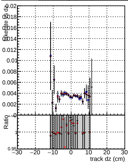
DOM mkFit5 XiMinusNOPUold-lowpt DOM mkFit5 XiMinusNOPUnewDefault5 DOM mkFit5 XiMinusNOPUnewDefault5 specPLeSS3
