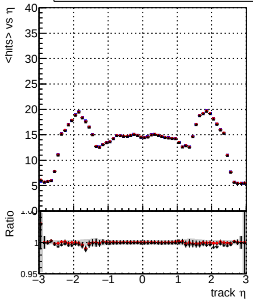
mean hits — DQM_mkFit5_XiMinusNOPUold-lowpt — DQM_mkFit5_XiMinusNOPU_newDefault5 — DQM_mkFit5_XiMinusNOPU_NEWdefault_specPless3
