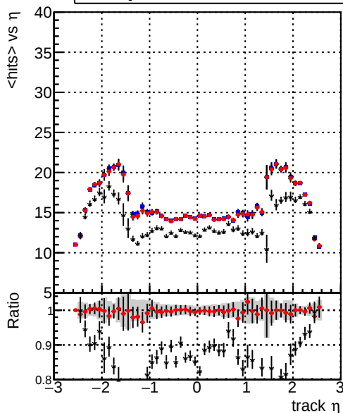
mean hit — DQM_mkFit5_XiMinusNOPUold-lowpt — DQM_mkFit5_XiMinusNOPU_newDefault5 — DQM_mkFit5_XiMinusNOPU_NEWdefault_specLess3
