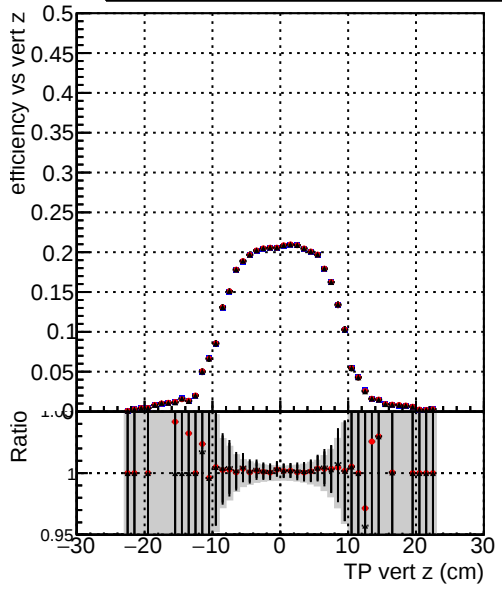
Efficiency vs vert z — DQM_mkFit5_XiMinusNOPUold-lowpt — DQM_mkFit5_XiMinusNOPU_newDefault5 — DQM_mkFit5_XiMinusNOPU_NEWdefault_specPless3
