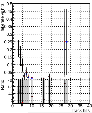
Fake rate vs hit DQM_mkFit5_XiMinusNOPUold-lowpt DQM_mkFit_XiMinusNOPU_newDefault5 DQM_mkFit_XiMinusNOPU_NEWdefault_specPLeSS3
