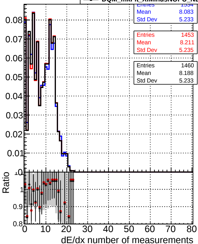
— DQM_mkFit5_XiMinusNOPUold-lowpt — DQM_mkFit5_XiMinusNOPU_newDefault5 — DQM_mkFit5_XiMinusNOPU_NEWdefault_specPLess3
