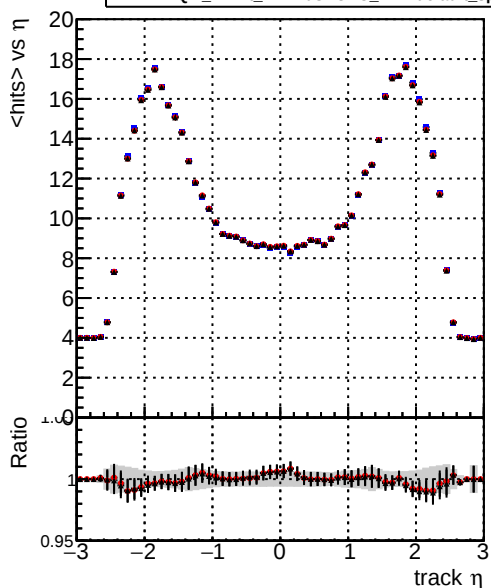
mean hit — DQM_mkFit5_XiMinusNOPUold-lowpt — DQM_mkFit5_XiMinusNOPU_newDefault5 — DQM_mkFit5_XiMinusNOPU_NEWdefault_specPless3
