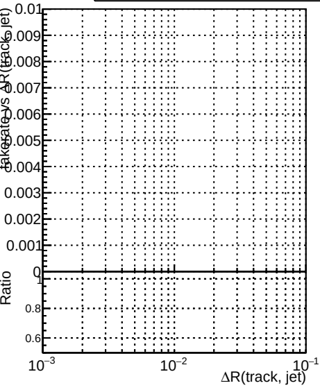
Fake rate vs \Delta R(\text{track, jet}) DQM_mkFit5_XiMinusNOPUold-lowpr DQM_mkFit5_XiMinusNOPUnewDefault5 DQM_mkFit5_XiMinusNOPUnewDefault5_specPLess3
