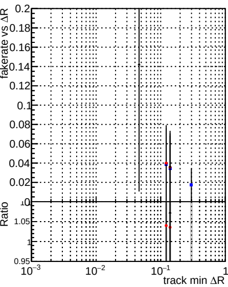
Fake rate vs \Delta R(\text{track, jet}) DQM_mkFit5_XiMinusNOPUold-lowpr DQM_mkFit5_XiMinusNOPUnewDefault5 DQM_mkFit5_XiMinusNOPUnewDefault5_specPLess3
