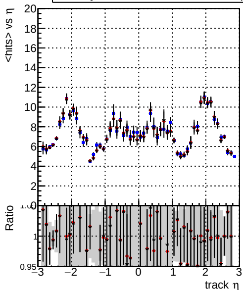
mean hit — DQM_mkFit5_XiMinusNOPUold-lowpt — DQM_mkFit5_XiMinusNOPU_newDefault5 — DQM_mkFit5_XiMinusNOPU_NEWdefault_specLess3
