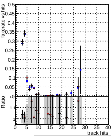
Fake rate vs hit Legend: DQM_mkFit5_XiMinusNOPUold-lowpt DQM_mkFit_XiMinusNOPU_newDefault5 DQM_mkFit_XiMinusNOPU_NEWdefault_specPLeSS3
