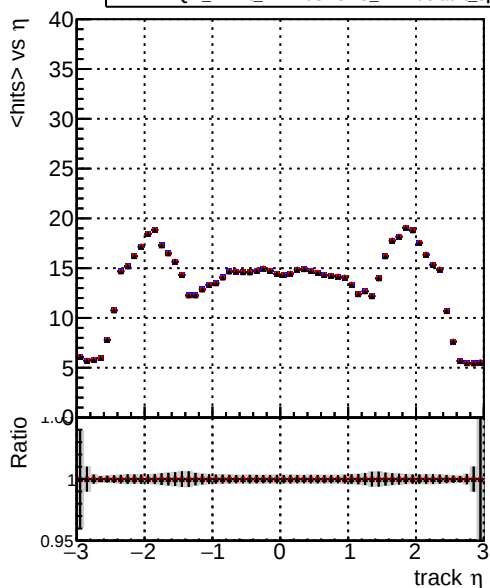
mean hits vs \eta — DQM_mkFit5_XiMinusNOPUold-lowpt — DQM_mkFit5_XiMinusNOPU_newDefault5 — DQM_mkFit5_XiMinusNOPU_NEWdefault_specPless3
