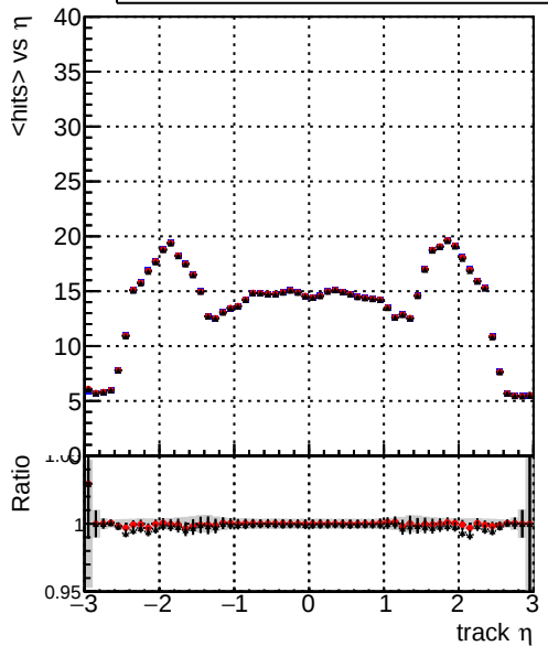
mean hit — DQM_mkFit5_XiMinusNOPUold-lowpt — DQM_mkFit5_XiMinusNOPU_newDefault5 — DQM_mkFit5_XiMinusNOPU_NEWdefault_specPLess3
