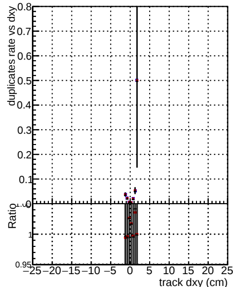
DOM mkFit5 XiMinusNOPUold-lowpt DOM mkFit5 XiMinusNOPUnewDefault5 DOM mkFit5 XiMinusNOPUnewDefault5 specPLess3
