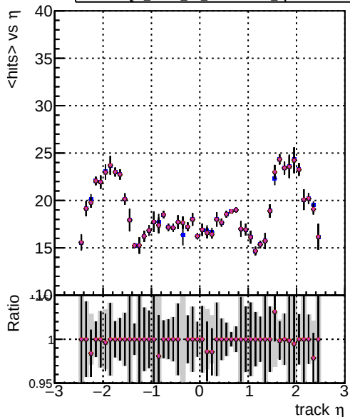
mean hit DQM mkFit TT NEWdefault specPless1 DQM mkFit TT NEWdefault specPless2 DQM mkFit TT NEWdefault specPless3 DQM mkFit TT NEWdefault specPless4
