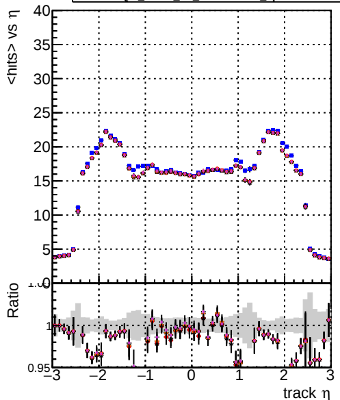
DQM mkFit TT NEWdefault specPless1 DQM mkFit TT NEWdefault specPless2 DQM mkFit TT NEWdefault specPless3 DQM mkFit TT NEWdefault specPless4
