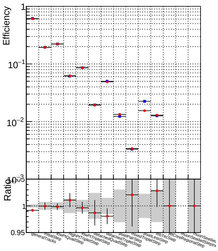
DQM_mkFit_TT_retrain DQM_mkFit_TTold
