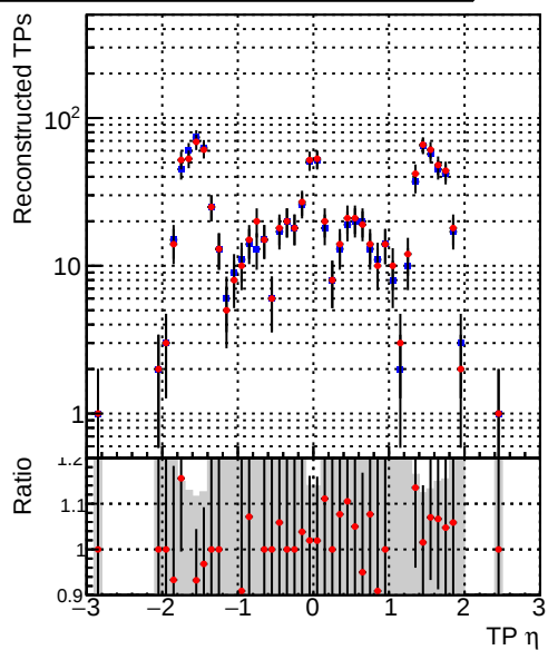
—●— DQM_mkFit_TT_retrain —●— DQM_mkFit_TTold
