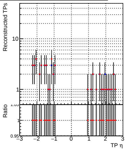
—●— DQM_mkFit_TT_retrain —●— DQM_mkFit_TTold
