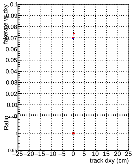
— DQM_mkFit_TT_retrain — DQM_mkFit_TTold
