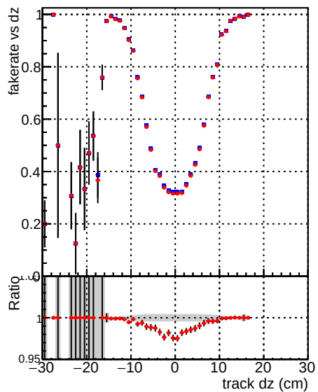
—●— DQM_mkFit_TT_retrain —●— DQM_mkFit_TTold
