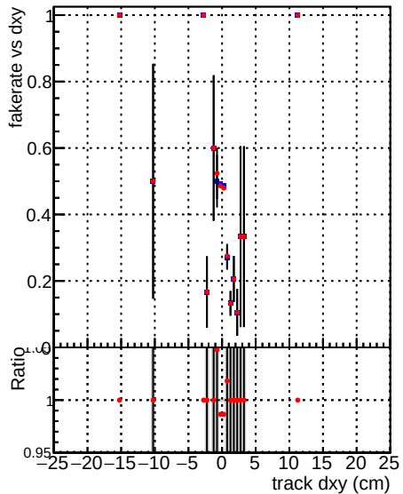
—●— DQM_mkFit_TT_retrain —●— DQM_mkFit_TTold
