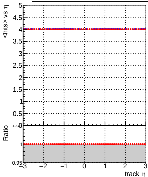
mean hits — DQM_mkFit_TT_retrain — DQM_mkFit_TTold
