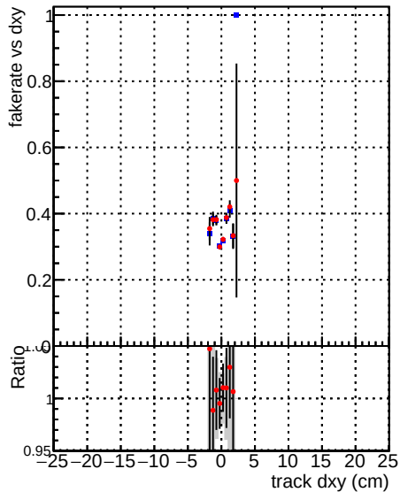
—●— DQM_mkFit_TT_retrain —●— DQM_mkFit_TTold
