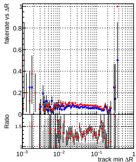
—●— DQM_mkFit_TT_retrain —●— DQM_mkFit_TTold
