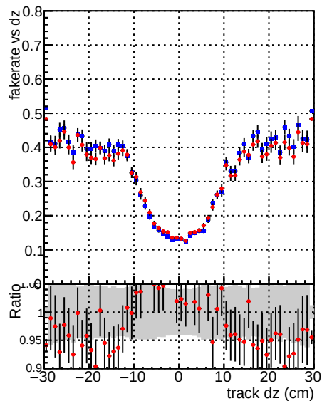
—●— DQM_mkFit_TT_retrain —●— DQM_mkFit_TTold
