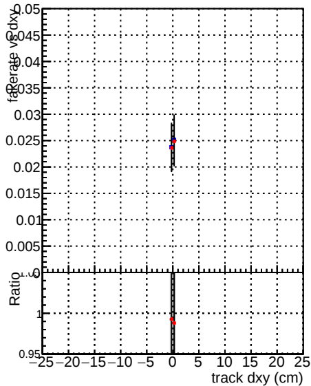
—•— DQM_mkFit_TT_retrain —•— DQM_mkFit_TTold
