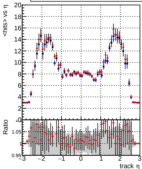
— DQM_mkFit_TT_retrain — DQM_mkFit_TTold mean hits
