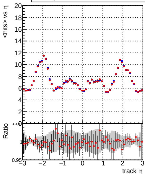
mean hit — DQM_mkFit_TT_retrain — DQM_mkFit_TTold
