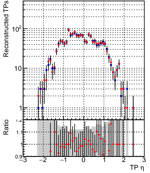
■ DQM_mkFit_TT_retrain ● DQM_mkFit_TTold
