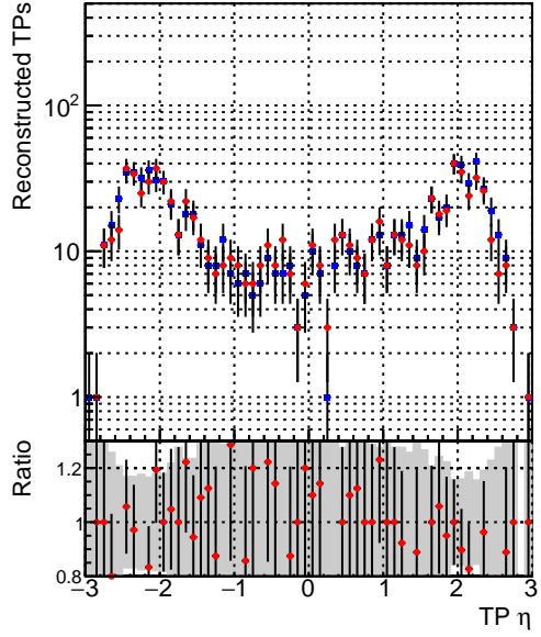
■ DQM_mkFit_TT_retrain ● DQM_mkFit_TTold
