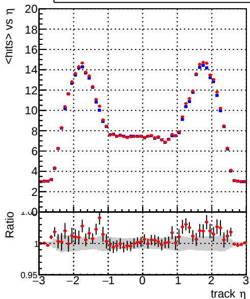
mean hit — DQM_mkFit_TT_retrain — DQM_mkFit_TTold
