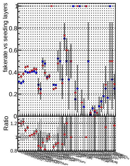
Fake rate vs. ◆ DQM mkFit TT_retrain ★ DQM mkFit TTold
