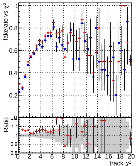
Fake rate vs. ◆ DQM mkFit TT_retrain ★ DQM mkFit TTold
