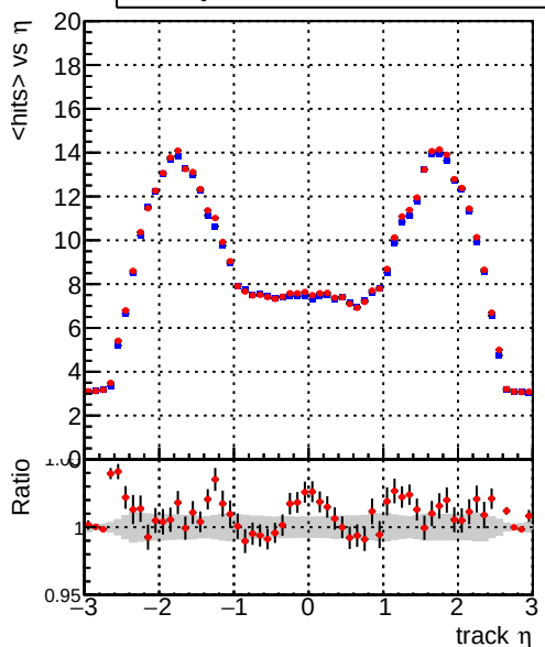
— DQM_mkFit_TT_retrain — DQM_mkFit_TTold mean hits
